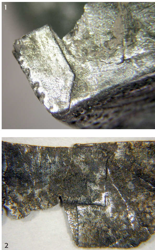
Obr. 7. Klecany II, hrob 22. Zjištěné způsoby spojů: 1 – na dně; 2 – nastřížení a spojení víčka. Foto A. Šilhová. — Abb. 7. Klecany II, Grab 22. Gefundene Verbindungsweisen: 1 – am Boden; 2 – Anschnitt und Verbindungsstellen des Deckels. Foto A. Šilhová.
