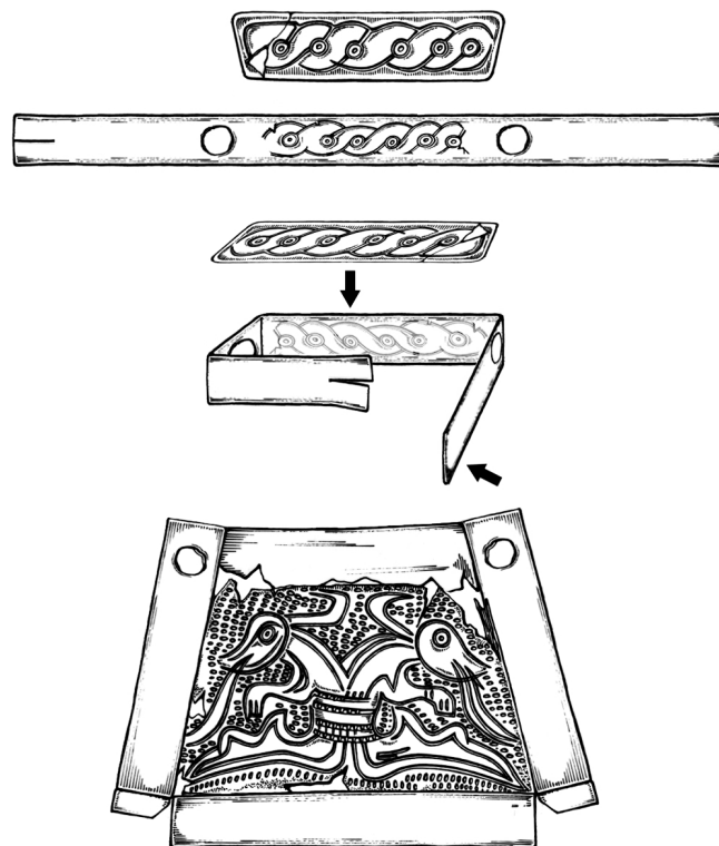
Obr. 8. Klecany II, hrob 22. Předpokládaný způsob výroby kaptorgy. Kresba I. Skokanová a A. Šilhová. — Abb. 8. Klecany II, Grab 22. Angenommene Herstellungsweise einer Kaptorgy. Zeichnung I. Skokanová und A. Šilhová.
