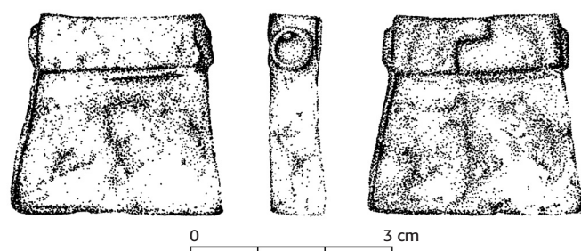
Obr. 18. Mělník. Kresba zachycuje dříve nepochopený a proto nedokumentovaný spoj na víčku kaptorgy a spoj zadní a boční stěny. Kresba L. Kos. — Abb. 18. Mělník. Die Zeichnung erfasst den früher unverständlichen und darum undokumentierten Verbindungspunkt auf dem Kaptorgendeckel und die Verbindung der Rück- und Seitenwand. Zeichnung L. Kos.
